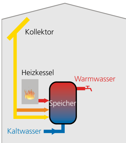
System B: 1-Speicher-System Vorwärmespeicher und Bereitschaftsspeicher in einem Speicher; geringerer Platzbedarf und geringe Wärmeverluste; geeignet, wenn bestehende Speicher ersetzt werden müssen.
